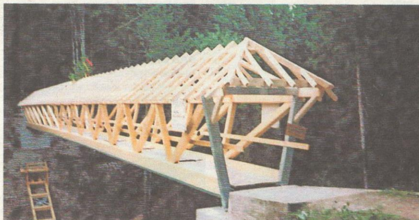
Die 42 Meter lange Badtöbeli-Brücke.
